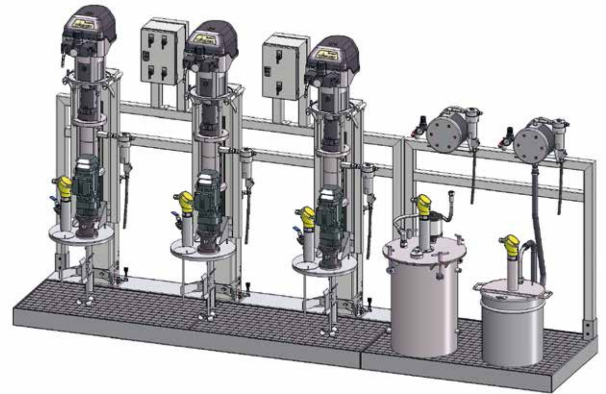
Zeichnung der fertigen Konstruktion.
